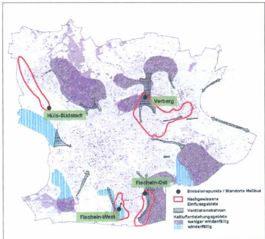
Abb. 7: Relevanz potentieller Kaltluftentstehungsgebiete und -leitbahnen in den vier Plangebieten Krefelds. Vier nächtliche Kaltluftausbreitungskampagnen (Tracer \text{SF}_6 ).
