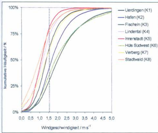
Abb. 6: Kumulative Häufigkeiten der Windgeschwindigkeiten im Krefelder Untersuchungsgebiet. (Basiszeitraum: 11/2001 bis 10/2002, Stundenmittelwerte).
