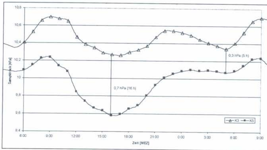
Abb. 5: Mittlerer Tagesgang des Dampfdrucks (hPa) am Stadt (K5)- und Umlandstandort (K3) in Krefeld (Basisgrundlage: Stundenmittelwerte; Messzeitraum: 11/2001 bis 10/2002).
