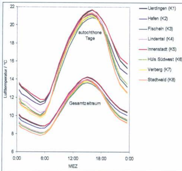
Abb. 3: Vergleich der durchschnittlichen Tagesgänge der Lufttemperatur im Gesamtzeitraum sowie an autochthonen Tagen im Krefelder Untersuchungsgebiet. Messzeitraum: 1. 11. 2001 bis 31. 10. 2002, Datengrundlage: Stundenmittelwerte.
