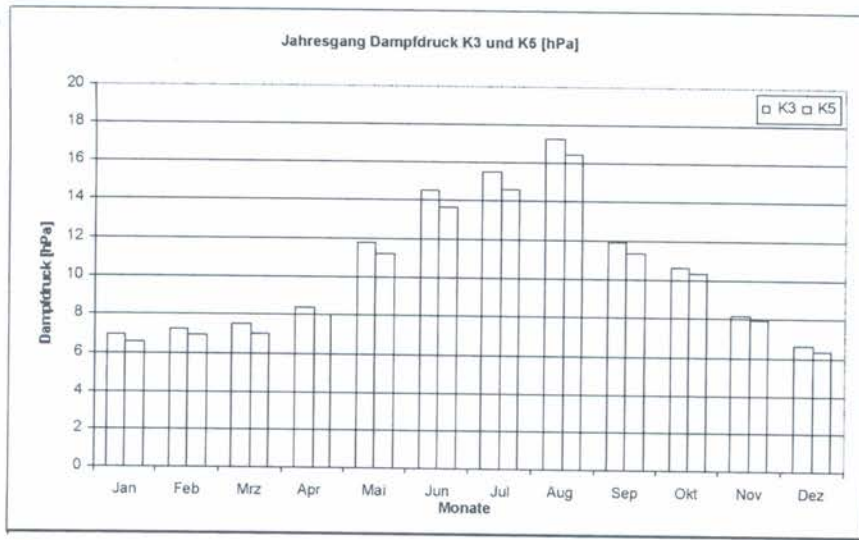
Abb. 4: Monatsmittelwerte des Dampfdrucks (hPa) am Stadt (K5)- und Umlandstandort (K3) in Krefeld (Basis: Stundenmittelwerte; 11/2001 bis 10/2002).
