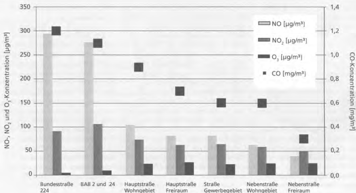
(9) Darstellung mittlerer Immissionskonzentrationen verschiedener kfz-bürtiger Spurenstoffe für unterschiedliche Straßentypen Gelsenkirchens. Datenbasis: Streckenabschnittsmittelwerte der lufthygienischen Profilmessfahrten vom 16.06.; 08.07.; 24.08.; 02.09.1999 jeweils zwischen 10.00 und 16.00 Uhr.
