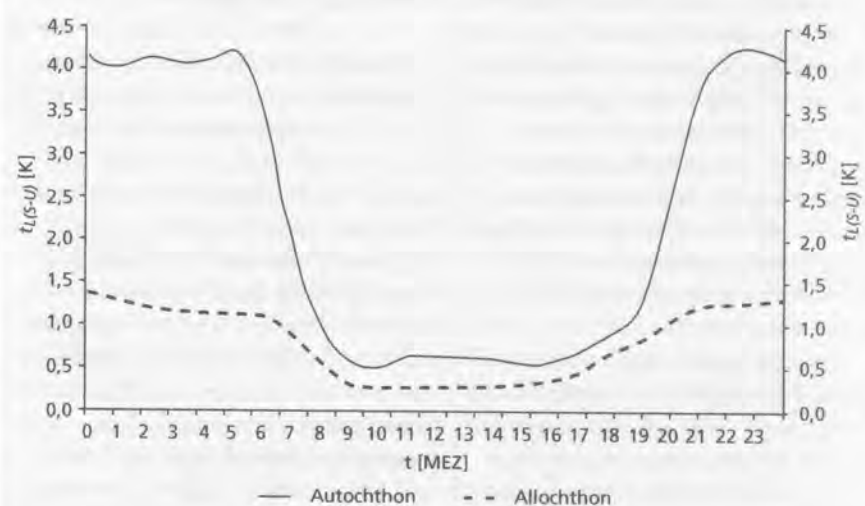
(2) Mittlerer Tagesgang der Lufttemperaturdifferenzen zwischen einer Stadt- (S) und einer Umlandstation (U) für autochthone und allochthone Wetterlagen der Messperiode 7/1995 bis 6/1996 in Köln.
