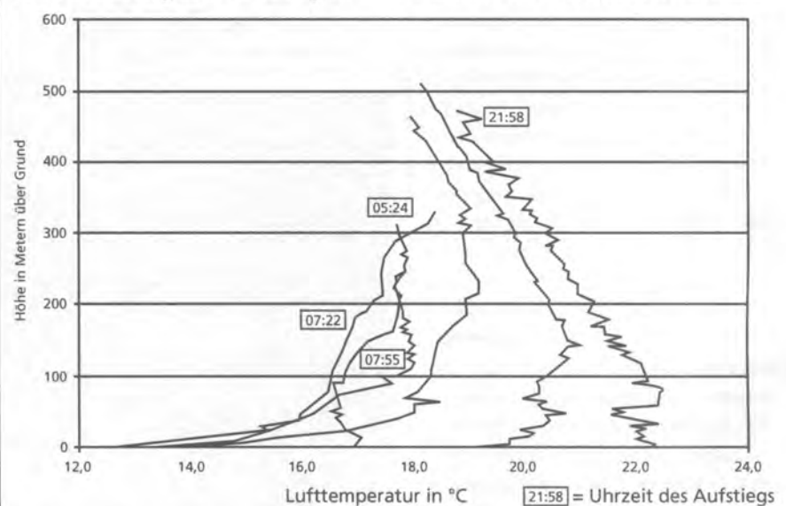
(7) Ausgewählte Vertikalprofile der Lufttemperatur in Gelsenkirchen. Datenbasis: nächtliche Fesselballonsondierungen (17./18.06.1999) im Nordsternpark (Station 5). Quelle: W. Kuttler, A. Kreft, S. Schaefers, A.-B. Barlag: Gesamtstädtische Klimaanalyse Gelsenkirchen, Endbericht, durchgeführt im Auftrag der Stadt Gelsenkirchen, Umweltamt (unveröffentlicht), Essen 2000, verändert
