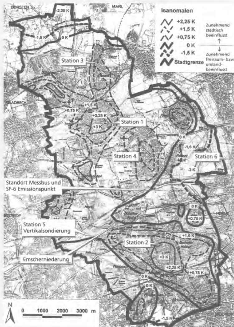
(5) Mess-Standorte und Verteilung der bodennahen Lufttemperaturdifferenzen (K) bezogen auf den Durchschnittswert von drei strahlungsnächtlichen Messfahrten innerhalb des Untersuchungszeitraums 01.11.1998 bis 31.10.1999 in der Stadt Gelsenkirchen. Quelle: W. Kuttler, A. Kref, S. Schaefers, A.-B. Barlag: Gesamtstädtische Klimaanalyse Gelsenkirchen, Endbericht, durchgeführt im Auftrag der Stadt Gelsenkirchen, Umweltamt (unveröffentlicht), Essen 2000, verändert
