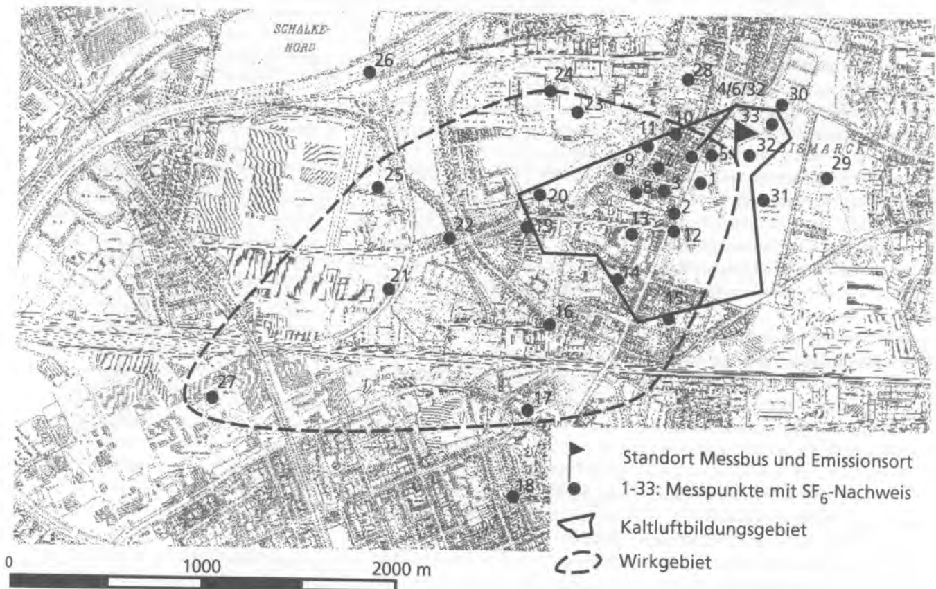
(8) Kaltluftausbreitungskampagne mittels Schwefelhexafluorid ( SF_6 ) in Gelsenkirchen in der Nacht vom 04./05.11.1999. Quelle: W. Kuntler, A. Krefz, S. Schaefers, A.-B. Barlag: Gesamtstädtische Klimaanalyse Gelsenkirchen, Endbericht, durchgeführt im Auftrag der Stadt Gelsenkirchen, Umweltamt (unveröffentlicht), Essen 2000, verändert
